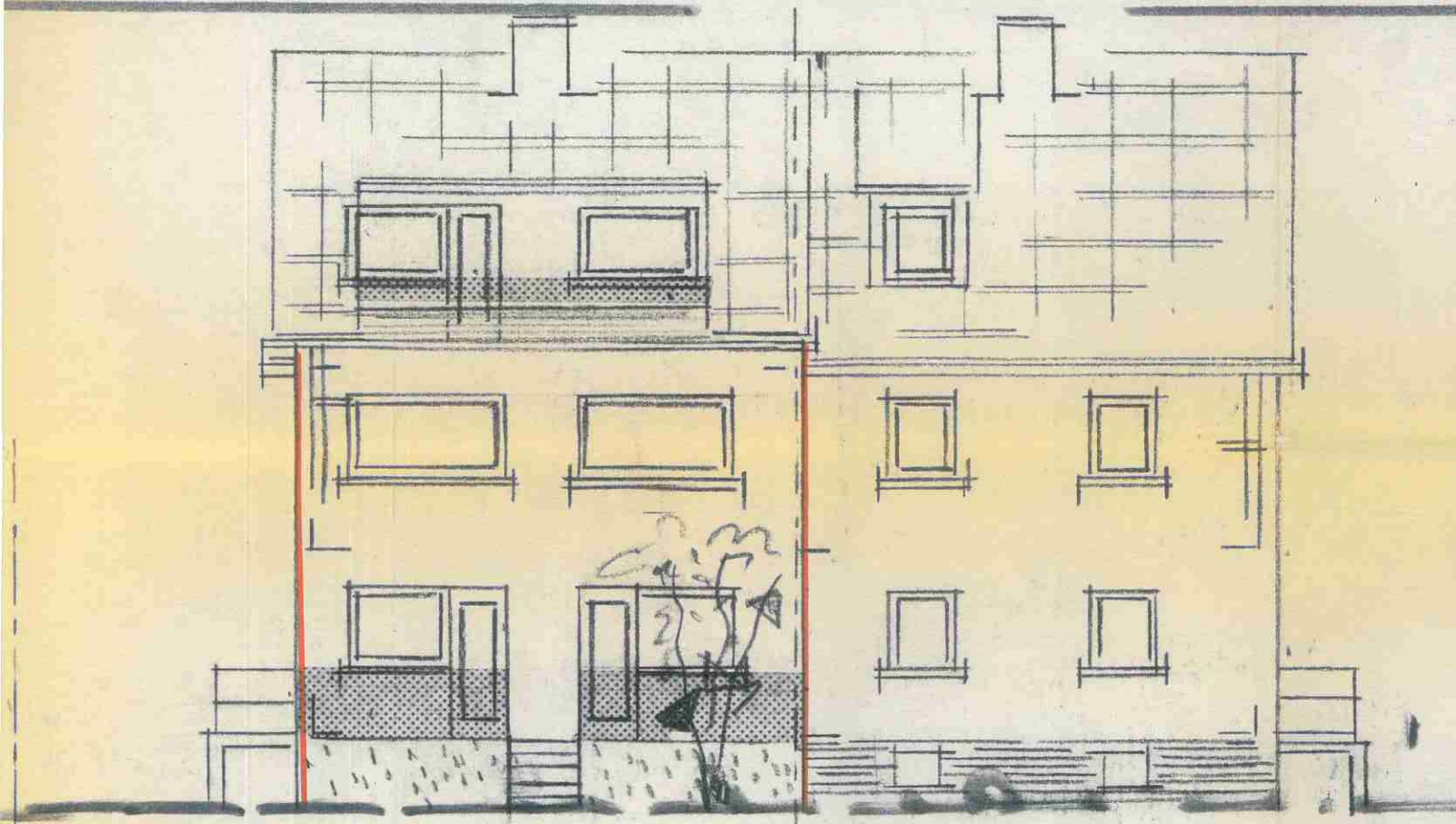
ANSICHT VORSEITE
