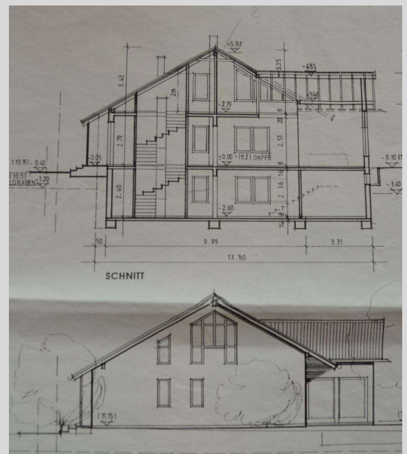
Schnitt, Ansicht
