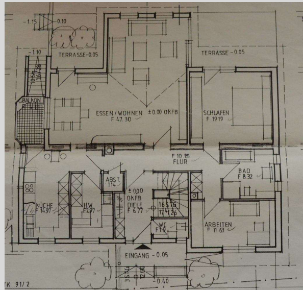
Erdgeschoss
