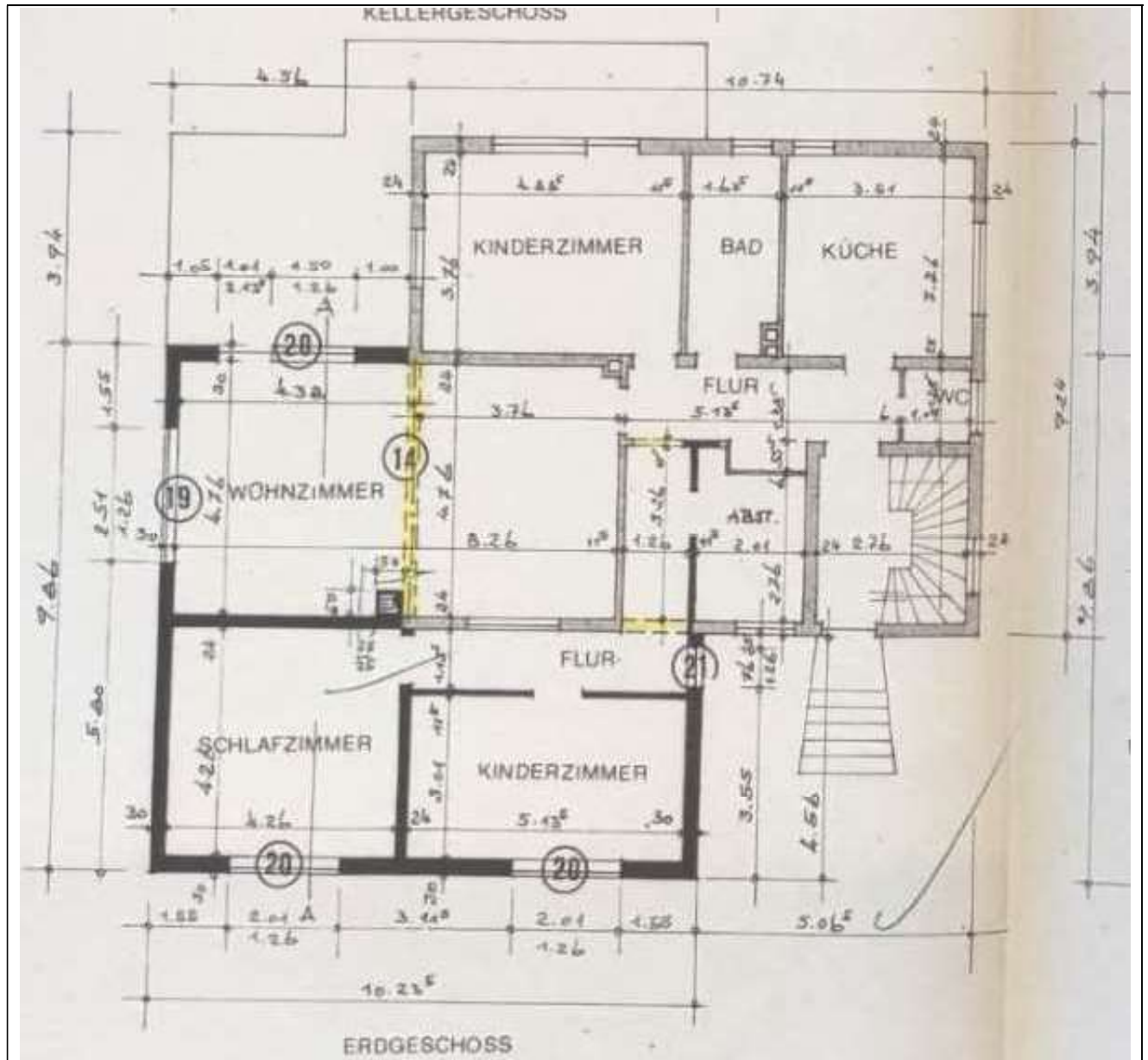
Anlage 5.1: Grundriss Erdgeschoss
