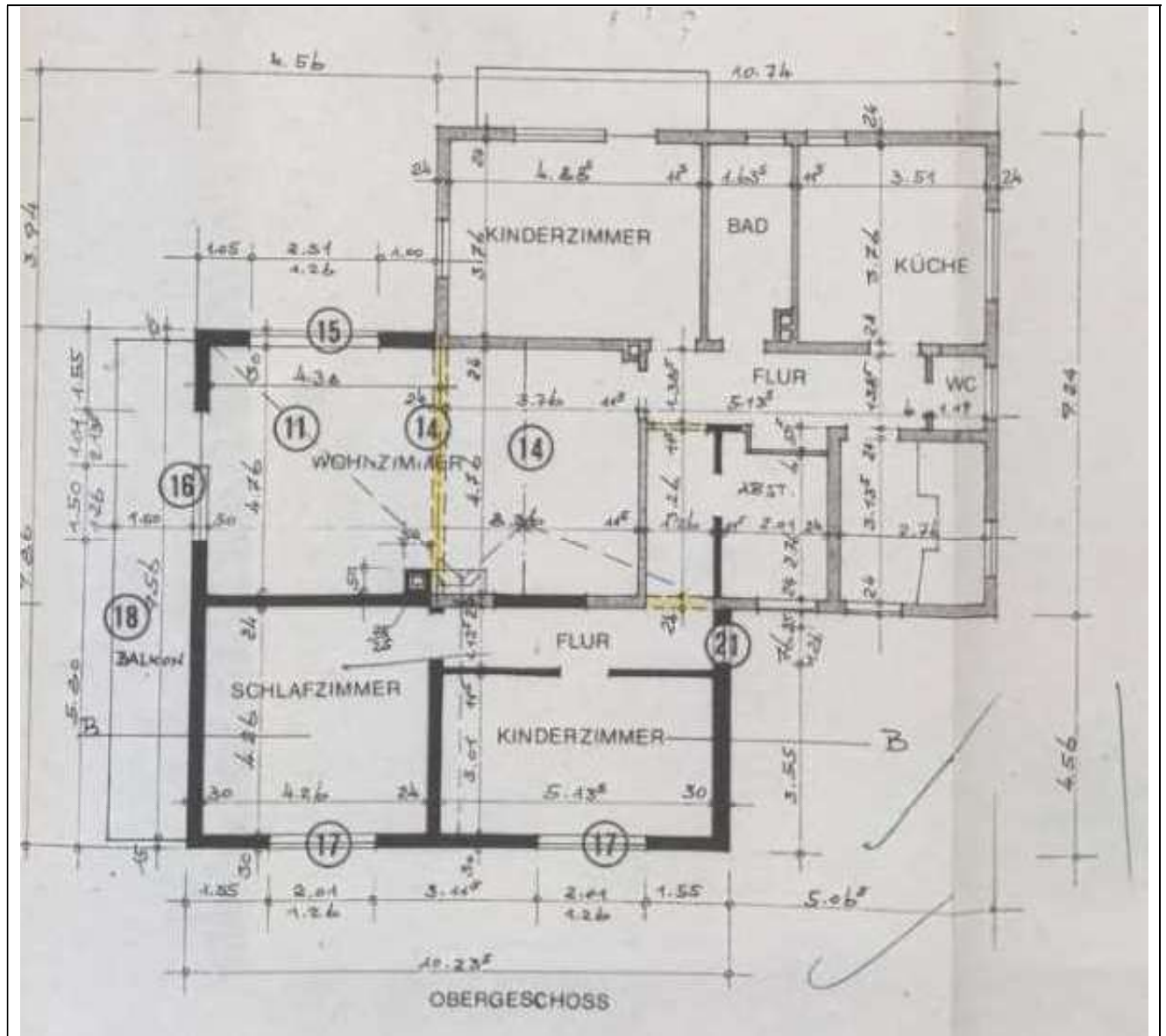
Anlage 5.3: Grundriss Obergeschoss
