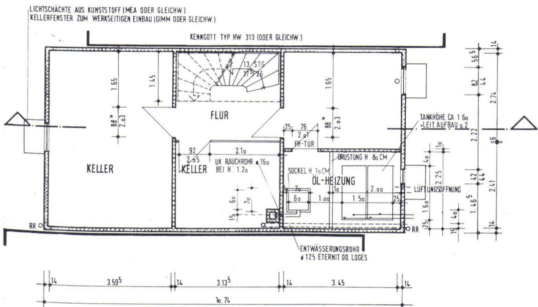
Kellergeschoss
