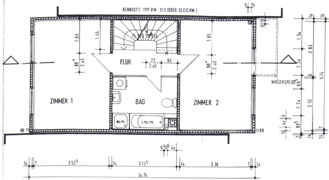
Obergeschoss
